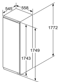
Maße in mm
