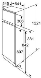
Maße in mm
