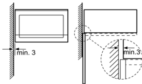
Maße in mm
